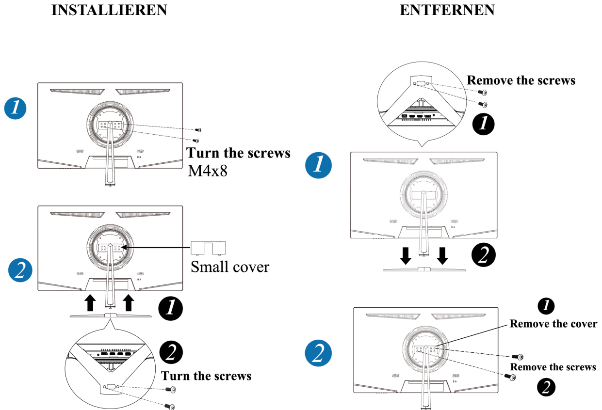
ABBILDUNG 1. INSTALLIEREN UND ENTFERNEN DES STÄNDERS
